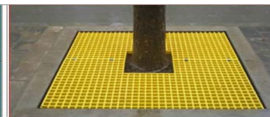
NEW! Size: 350x350mm., Tree Height: 40 cm., Thick: 30mm. คุณสมบัติ: ผลิตจากวัสดุคอมโพสิต FRP แข็งแรงทนทาน ใช้งานได้ยาวนาน น้ำหนักเบา ง่ายต่อการติดตั้ง ป้องกันการเกิดโรคโคนเน่า ป้องกันการเกิดโรคเหี่ยวตาย ป้องกันการเกิดโรคอื่นๆ
